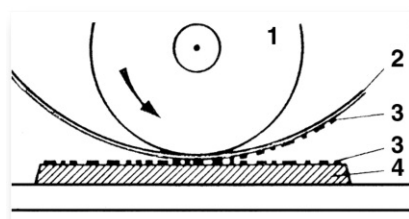
1 - přitlačný válec; 2 - papír; 3 - barva; 4 - tisková deska
